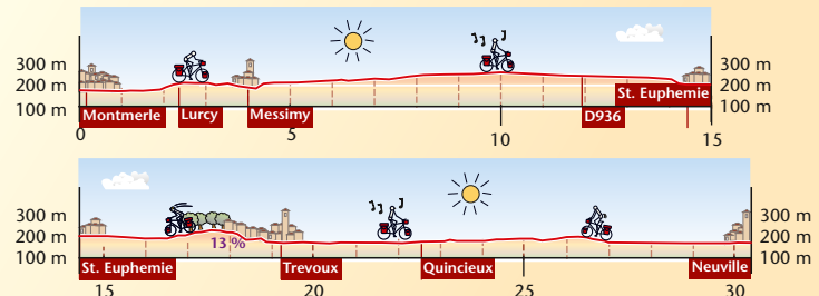
Routeprofiel route verharde weg Montmerle- Neuville
